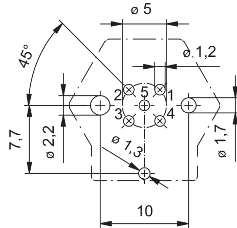
Leiterplatten-Layout
