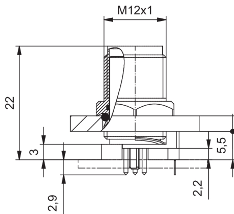
Frontplattenausschnitt
