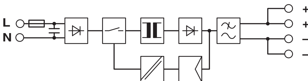
Schéma fonctionnel
