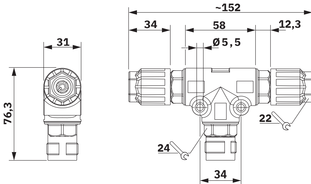
Maßzeichnung
