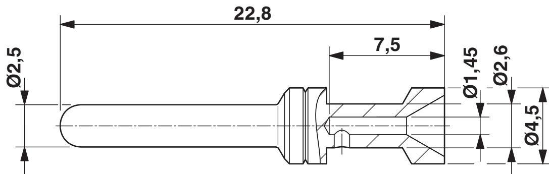
Dessin coté
