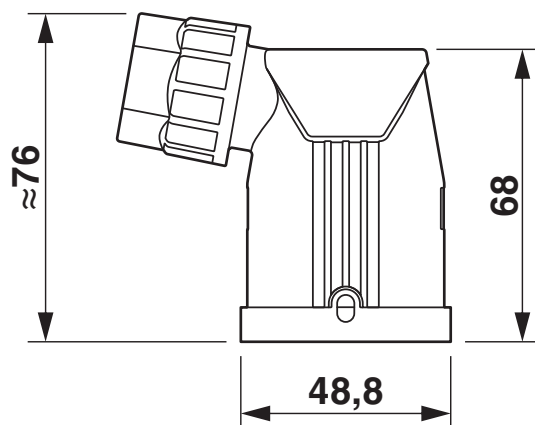
Esquema de dimensiones
