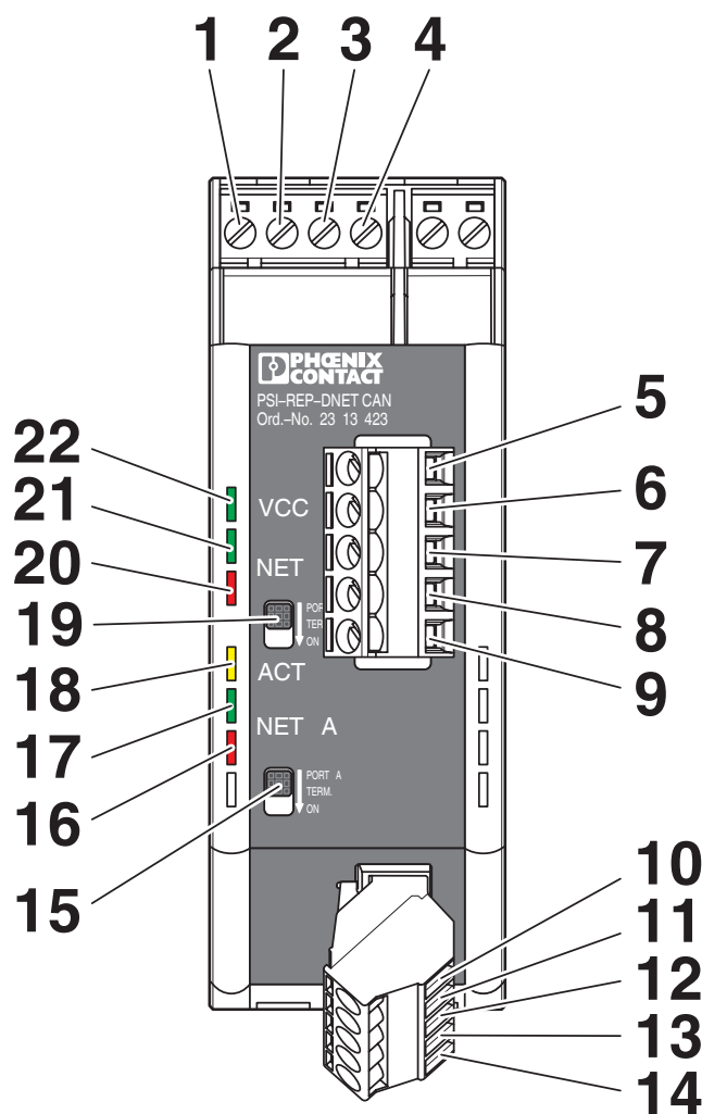
Dessin schématique
