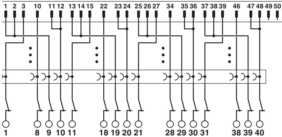
Diagrama eléctrico
