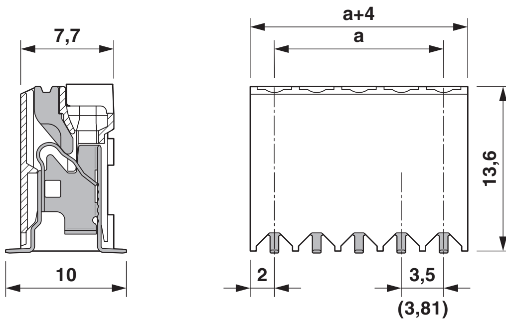
Maßzeichnung
