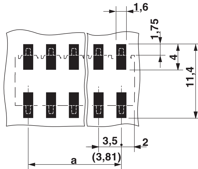
Bohrplan/Lötpadgeometrie
