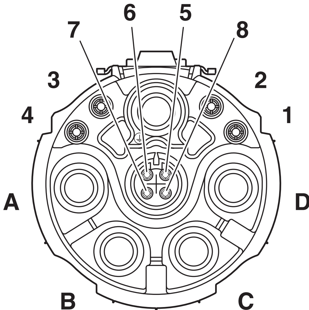
Schemazeichnung
