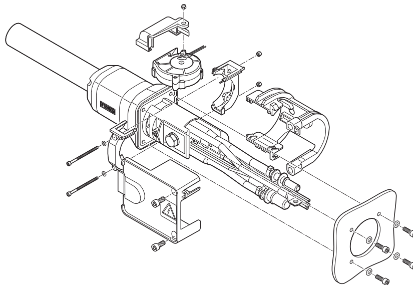
Plano esquemático
