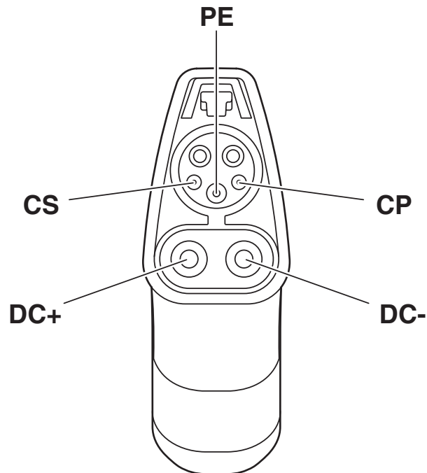
Plano esquemático
