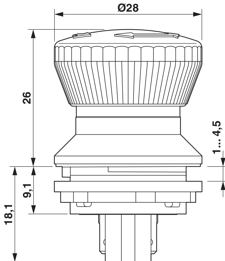
Maßzeichnung
