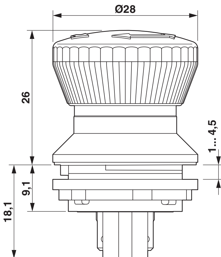
Dessin coté
