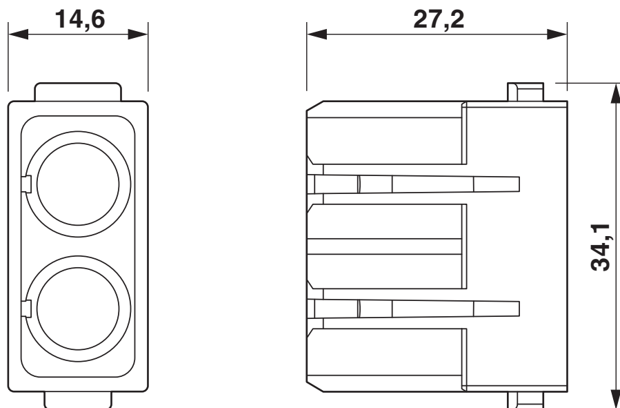
Dessin coté
