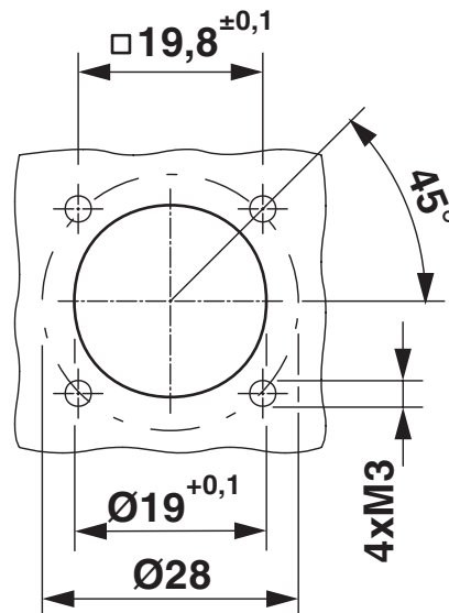
Maßzeichnung
