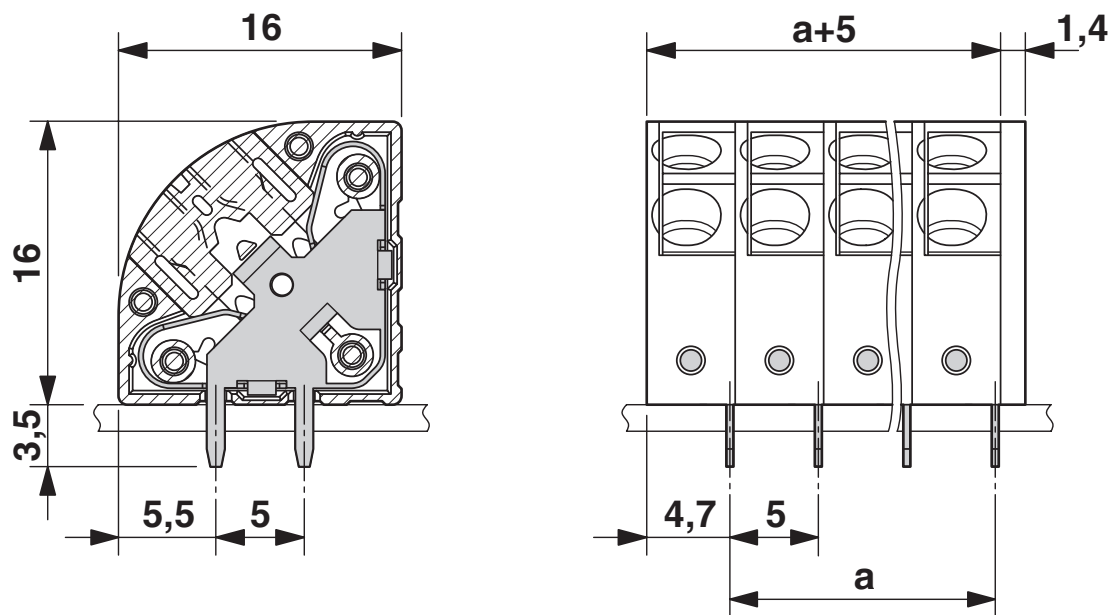
Dessin coté
