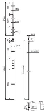
Maßbild HVI 23 L6M SR4700 IP RFS2500
