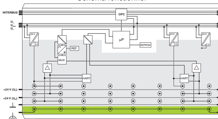
Schéma fonctionnel
