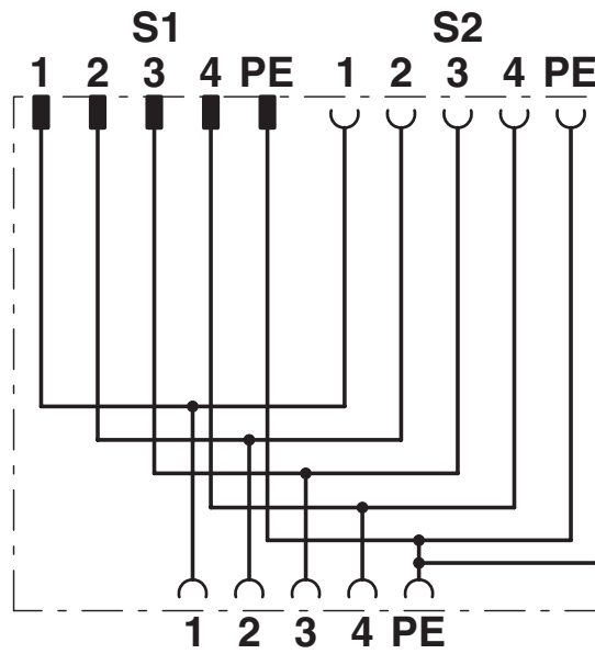
Schaltplan
