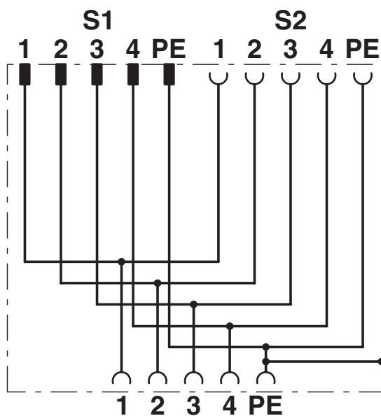
Diagrama eléctrico
