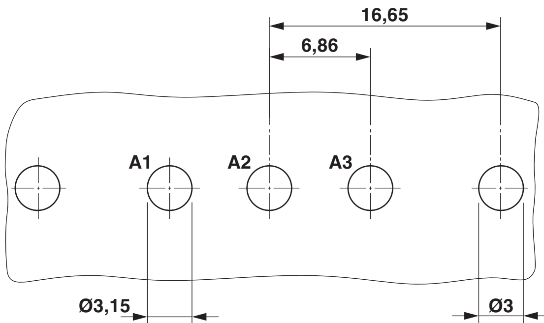
Esquema de taladros
