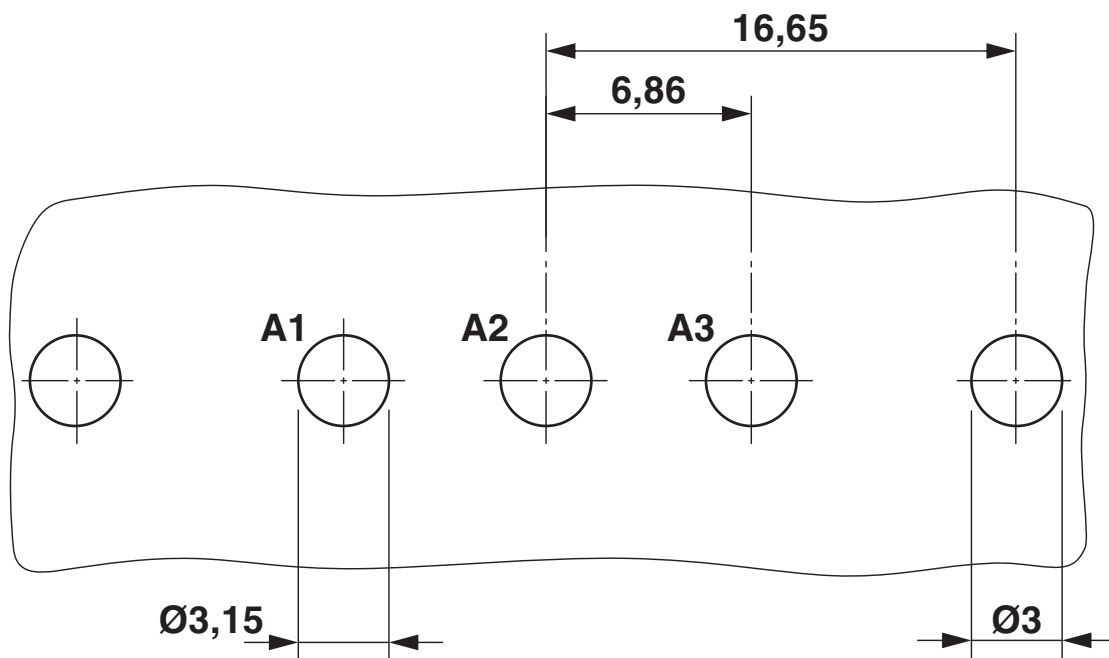
Gabarit perçage / géom. pastille soudage
