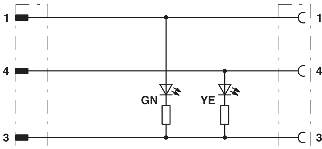
Disposition des contact des connecteurs mâles M8 / femelles M12
