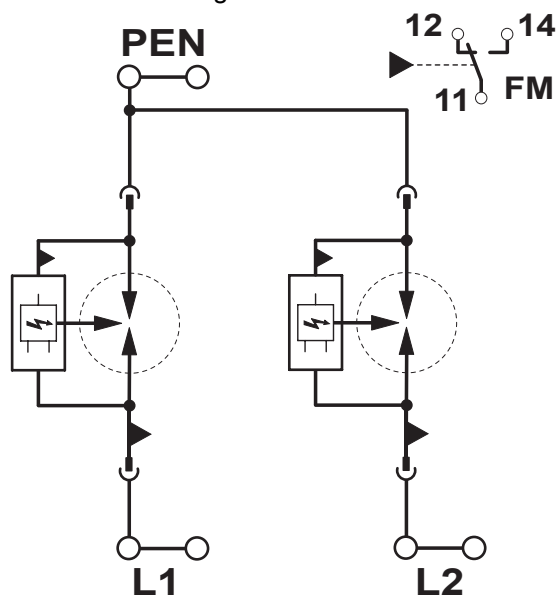
Diagrama eléctrico
