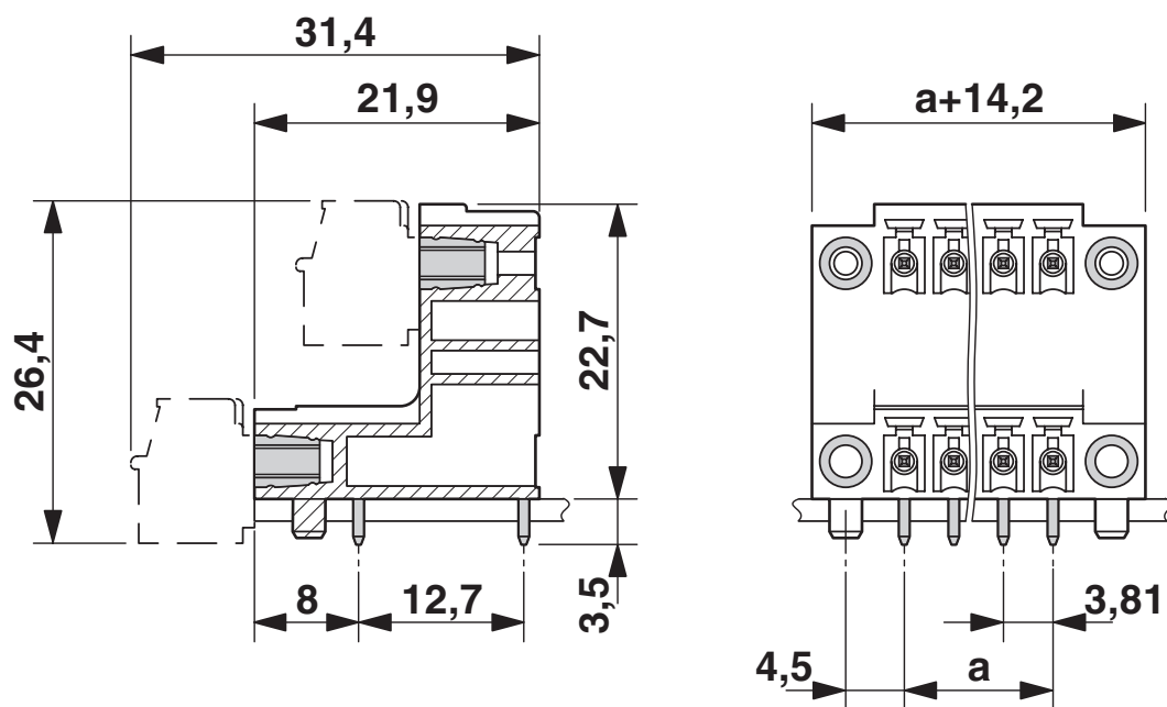
Dessin coté
