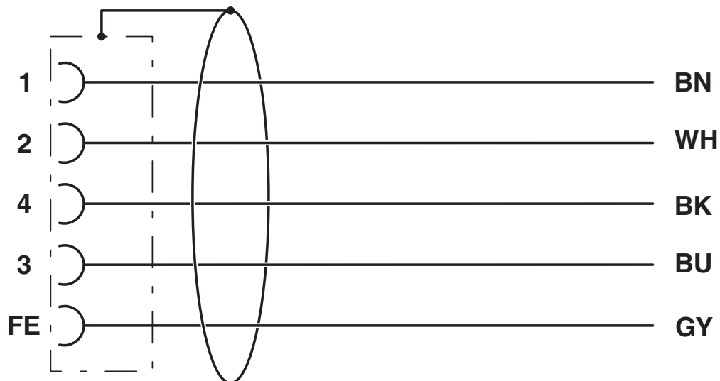
Diagrama eléctrico
