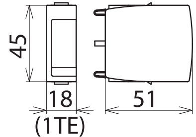
Maßbild DG MOD 600
