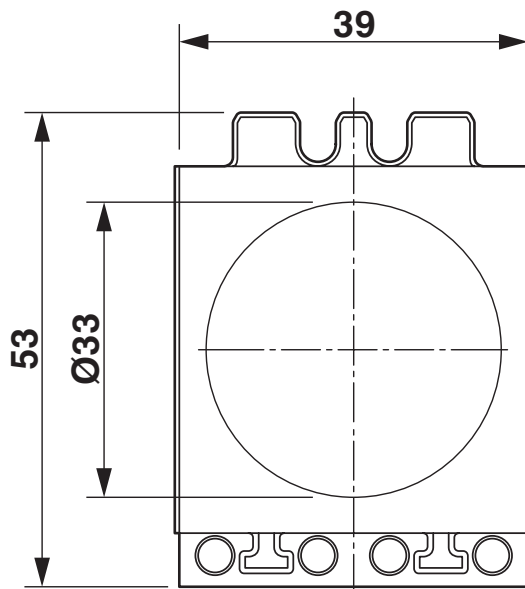
Dessin coté
