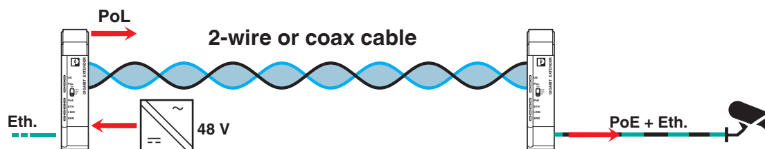
PoL-Versorgung des entfernten Extenders und PoE-Versorgung eines PoE-Endteilnehmers
