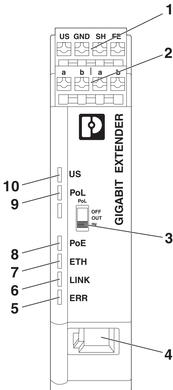
Schemazeichnung
