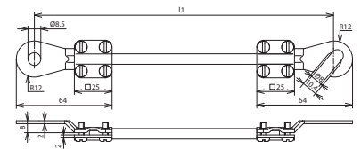
Maßbild EL16 L3.05M 1KSO 8.10 1KSG 8
