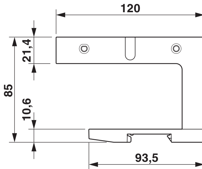
Maßzeichnung
