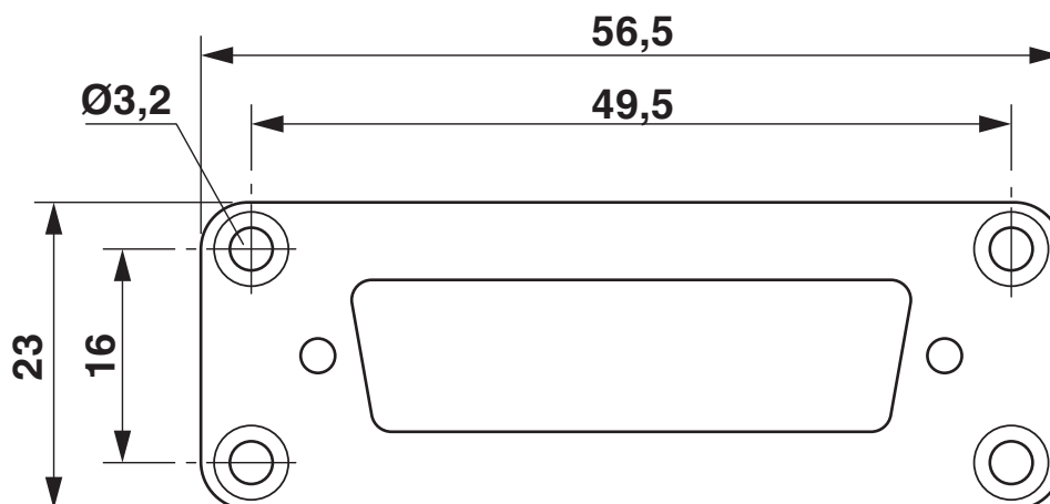
Maßzeichnung
