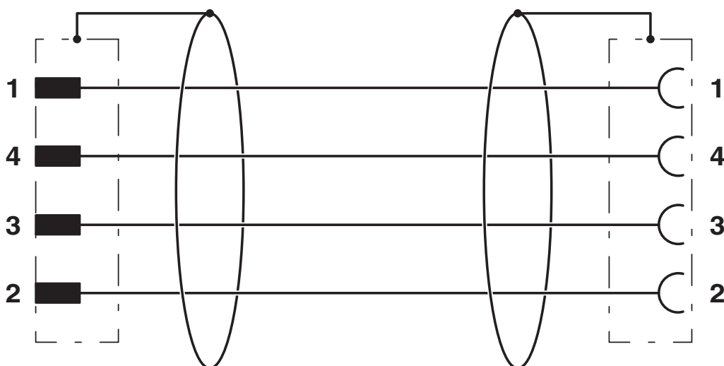
Ocupación de contactos del conector macho M12 y del conector hembra M12
