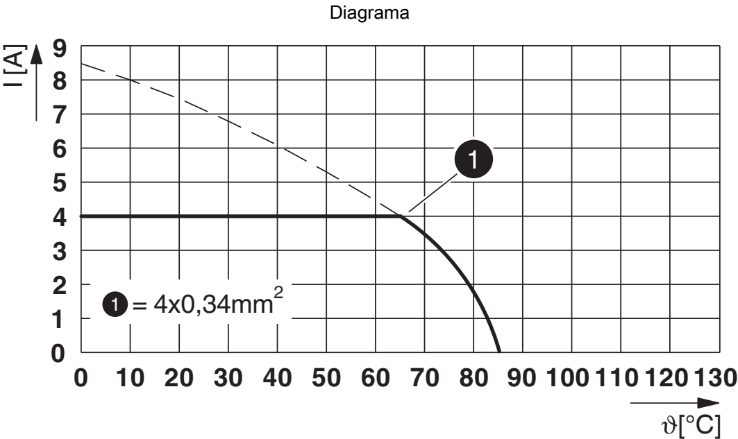
Diagrama eléctrico
