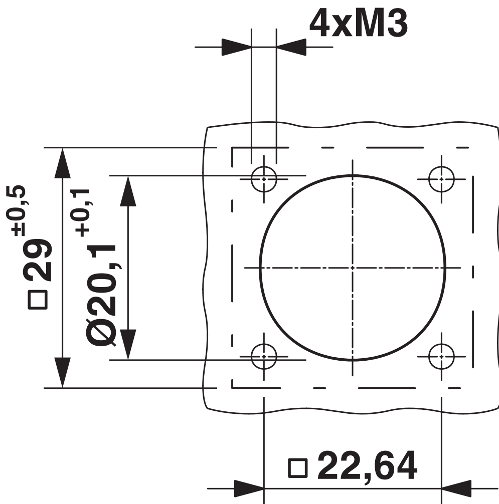
Maßzeichnung
