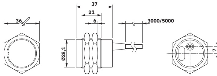
Maßzeichnung
