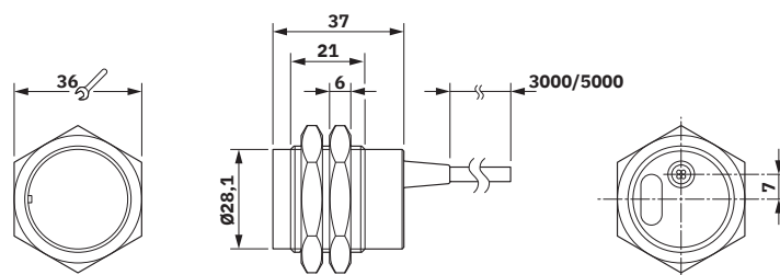
Dessin coté
