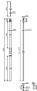
Maßbild HVI 23 L6M SR3200 IP FSP1000
