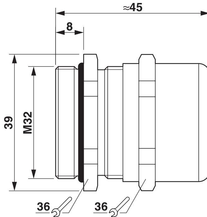
Maßzeichnung
