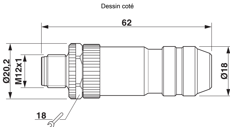
Connecteur mâle M12 x 1, droit, blindé
