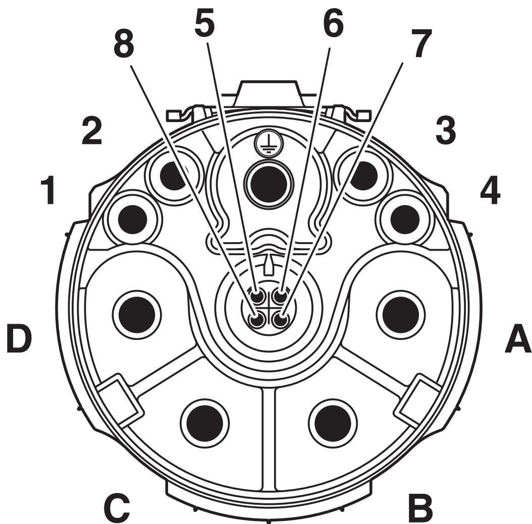
Plano esquemático
