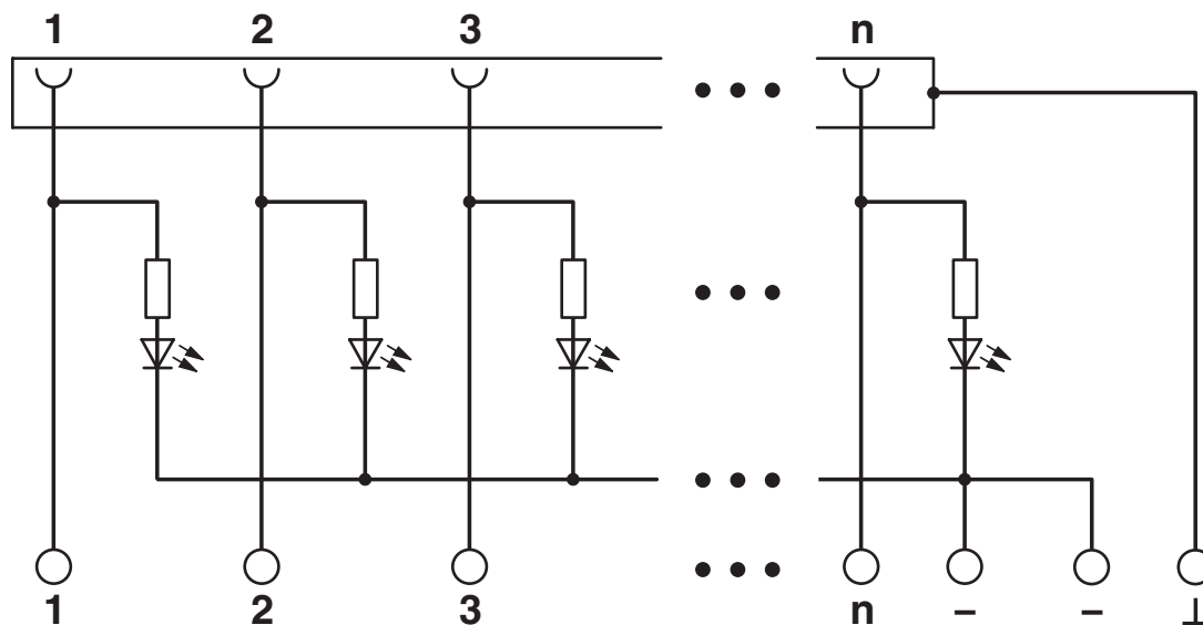
Diagrama eléctrico
