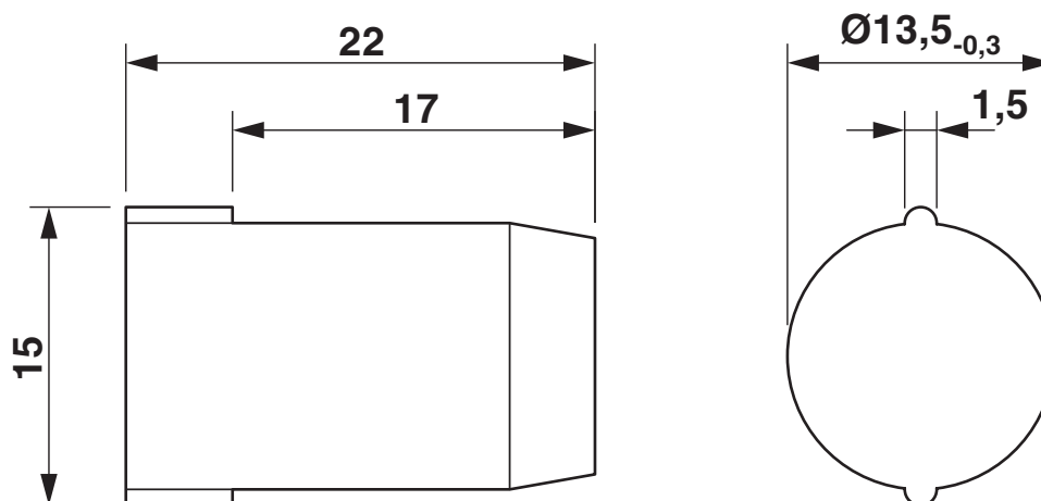
Maßzeichnung
