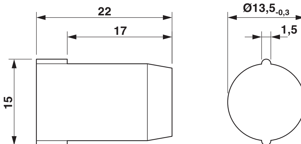
Dessin coté
