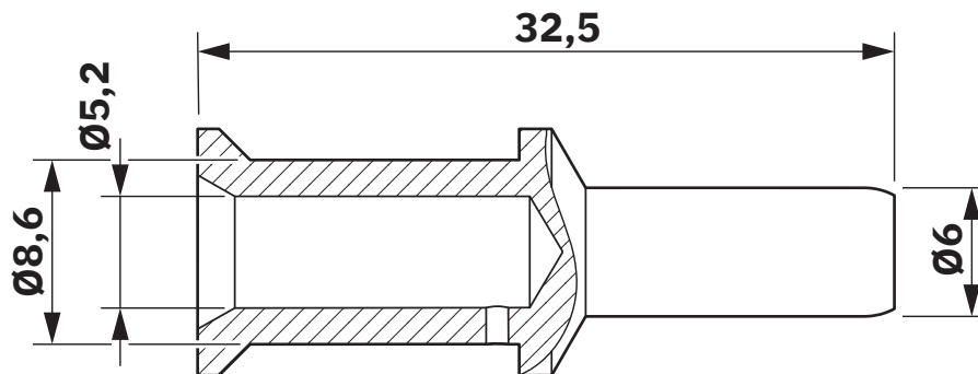
Dessin coté
