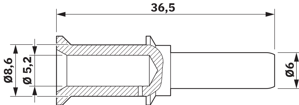
Dessin coté
