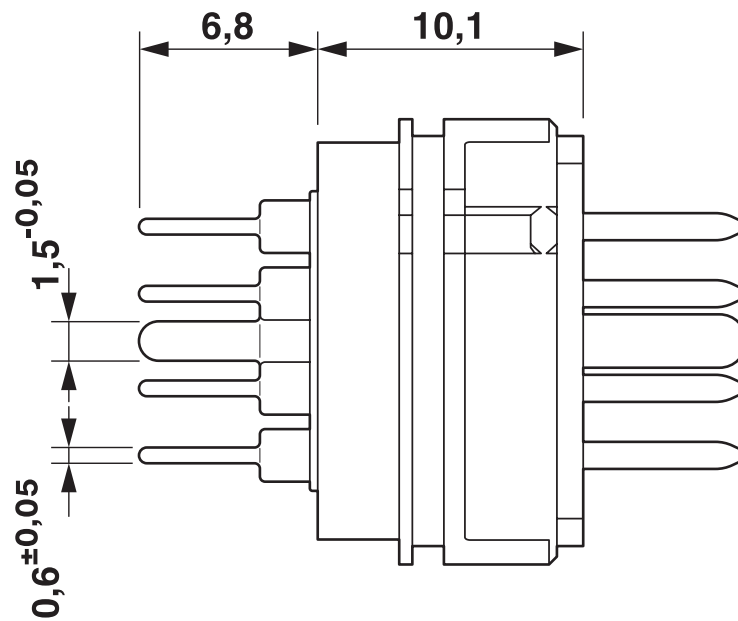
Maßzeichnung
