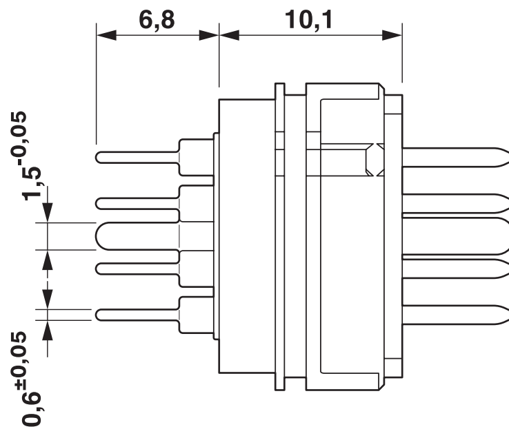
Dessin coté
