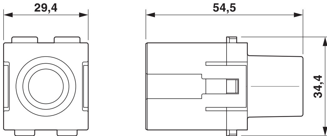
Maßzeichnung
