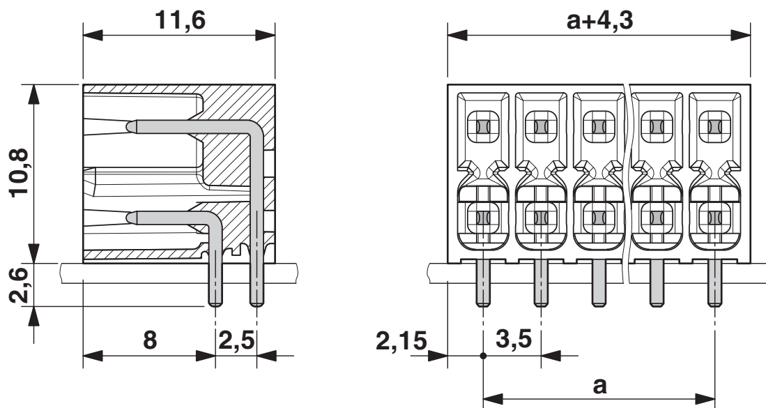
Schemazeichnung
