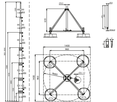
Maßbild FS T D50 1.8 8.0M AL VBS RA680
